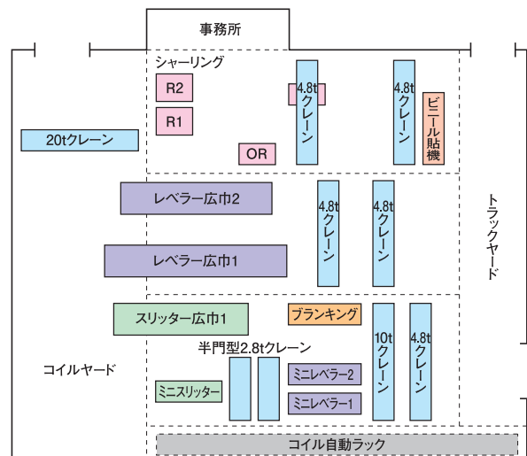
ブランク加工ライン
